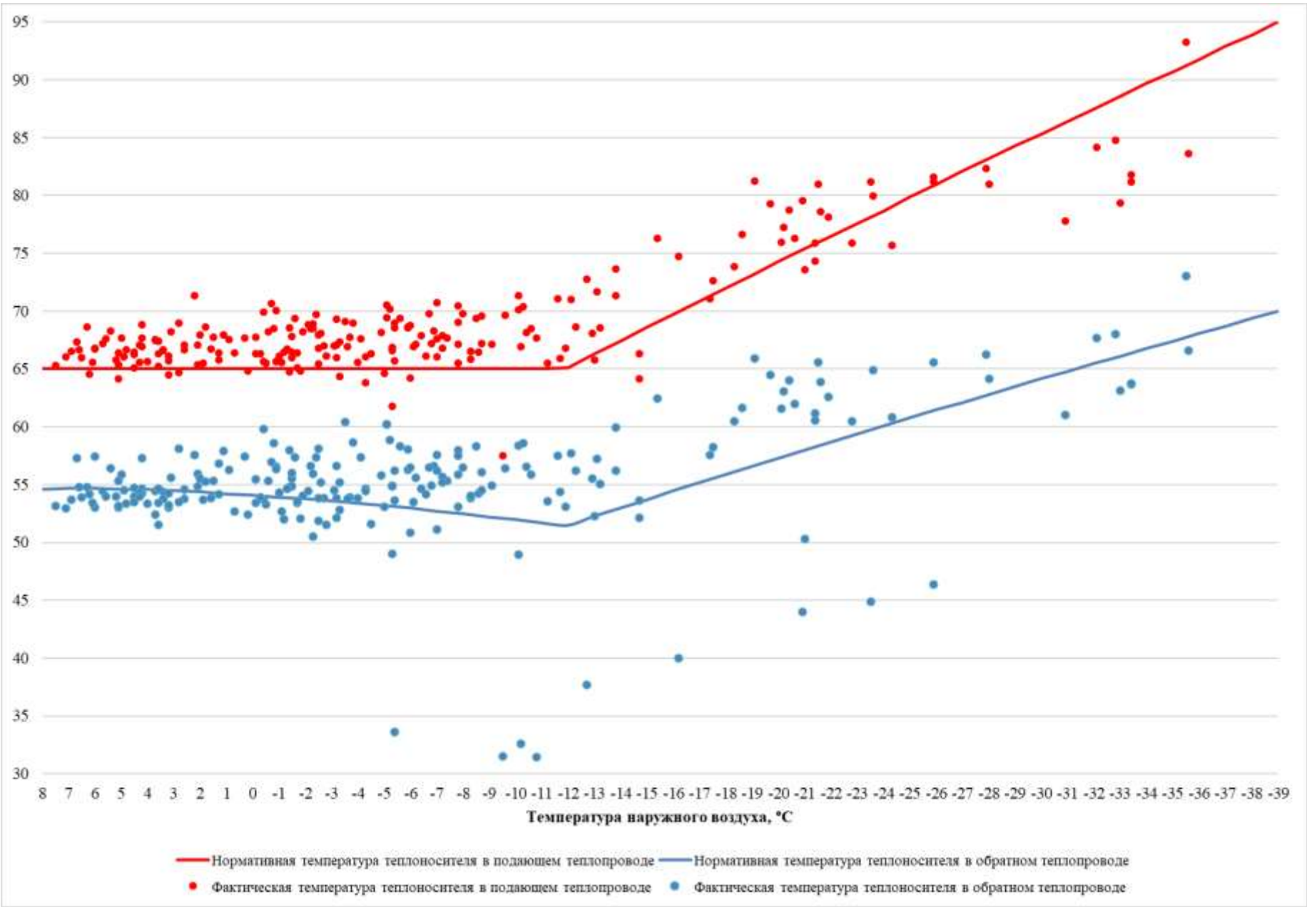
Рисунок 3.30 – Сравнение утвержденного и фактического температурных графиков за 2024 г. – Котельная №6
