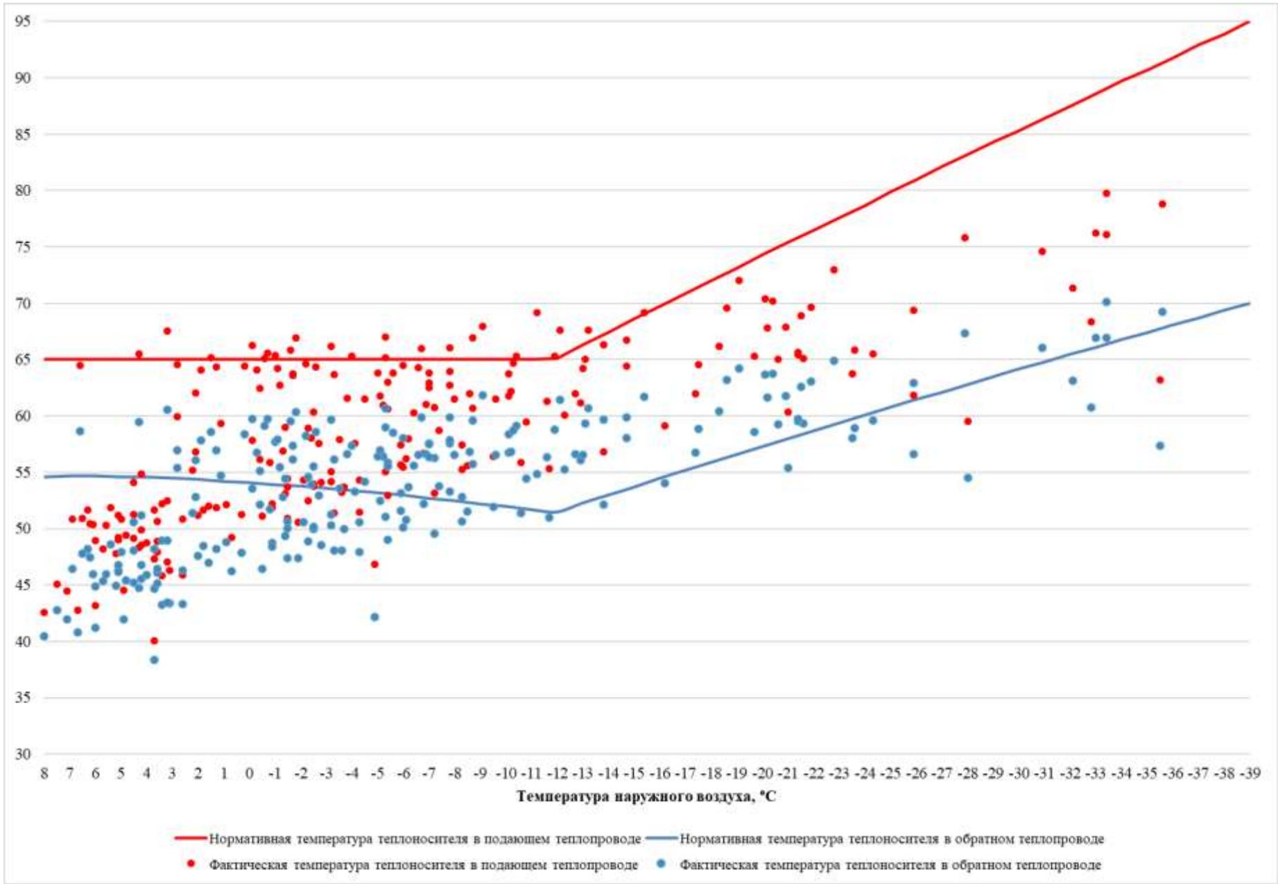
Рисунок 3.40 – Сравнение утвержденного и фактического температурных графиков за 2024 г. – Котельная школы №43
