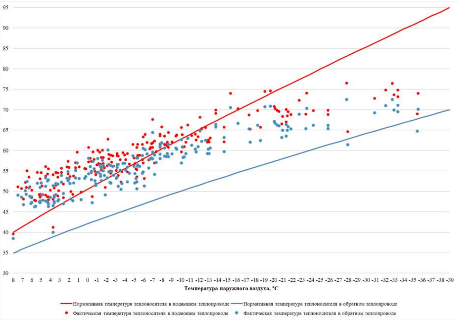
Рисунок 3.28 – Сравнение утвержденного и фактического температурных графиков за 2024 г. – Котельная №3 п. Абагур-Лесной
