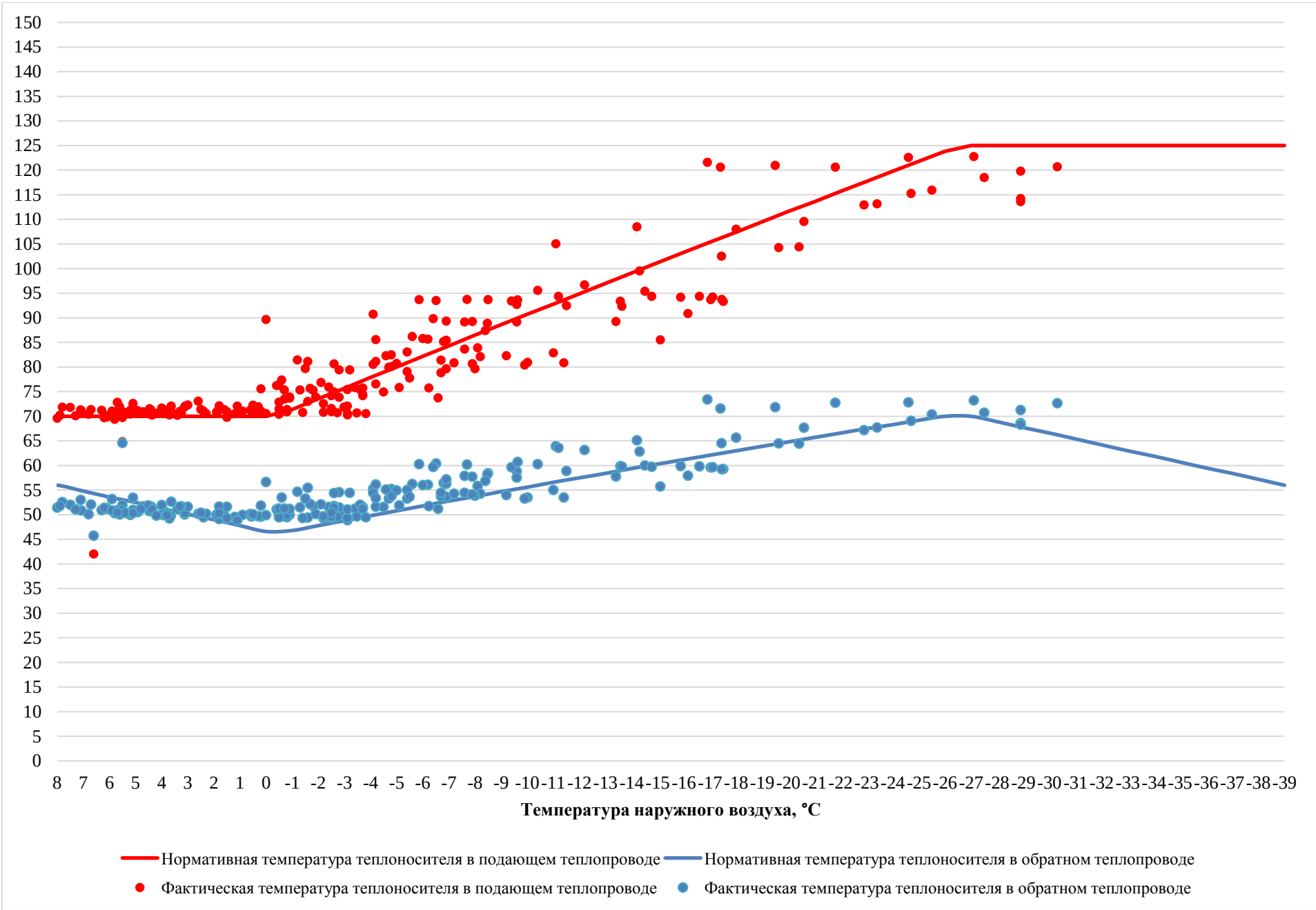
Рисунок 3.11 – Сравнение утвержденного и фактического температурных графиков за 2024 г. – Западный тепловывод ЗСТЭЦ
