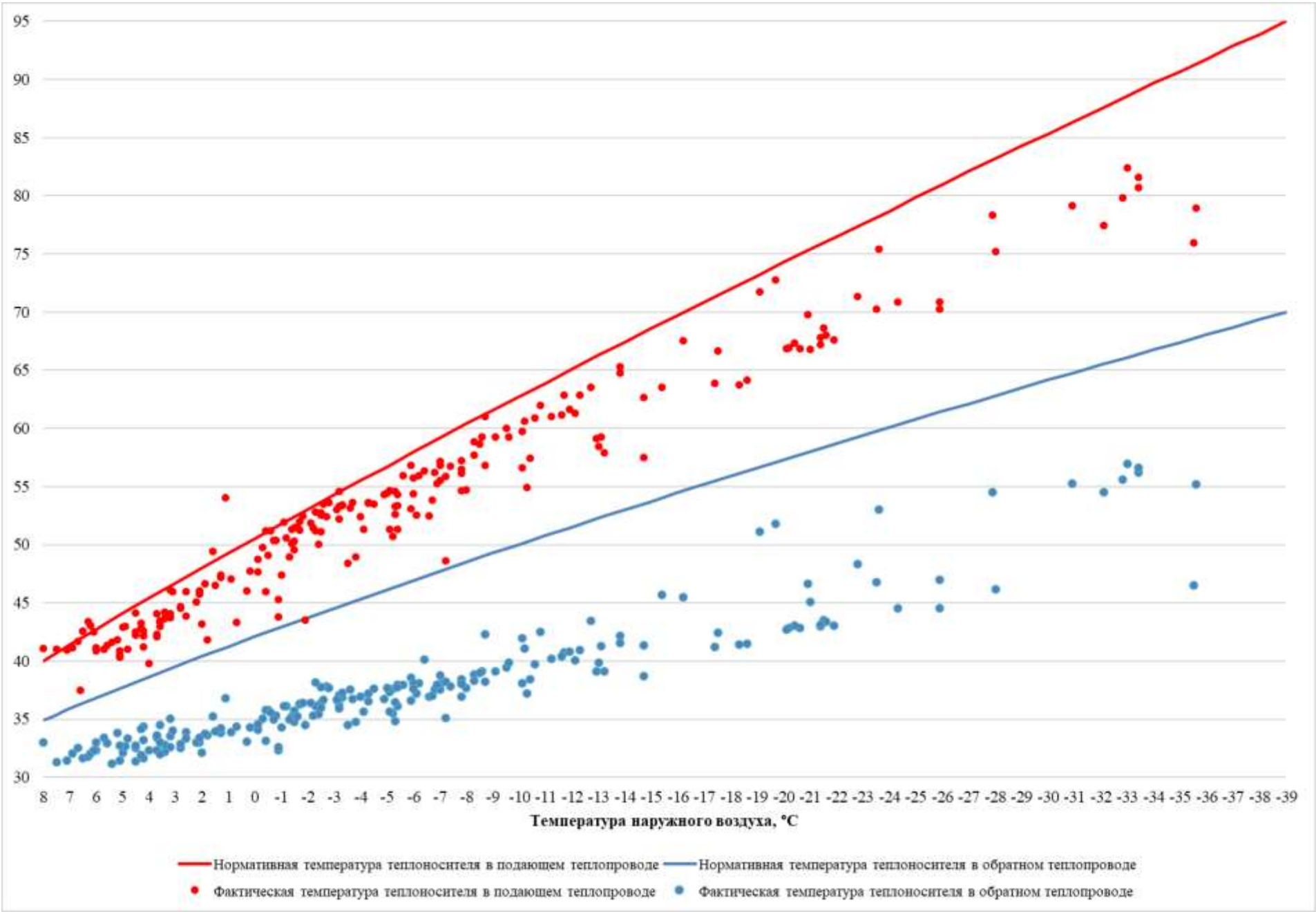
Рисунок 3.45 – Сравнение утвержденного и фактического температурных графиков за 2024 г. – Котельная «Кузнецкая крепость»
