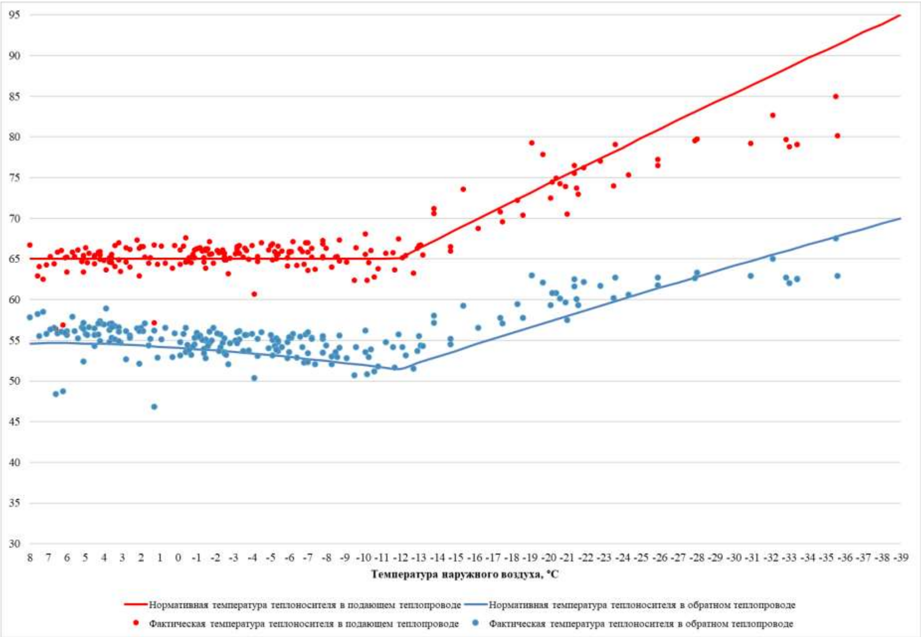
Рисунок 3.31 – Сравнение утвержденного и фактического температурных графиков за 2024 г. – Котельная №32 (БПОУ)
