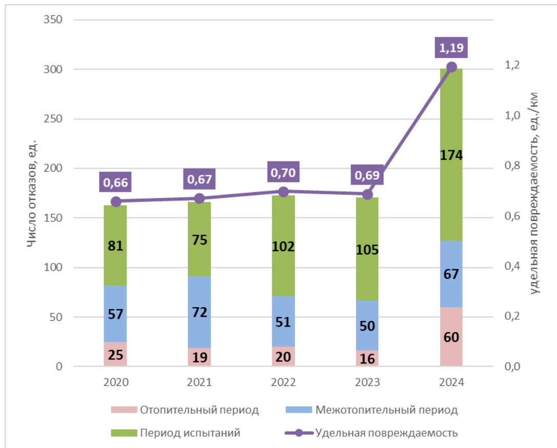
Рисунок 3.47 – Повреждаемость магистральных тепловых сетей
