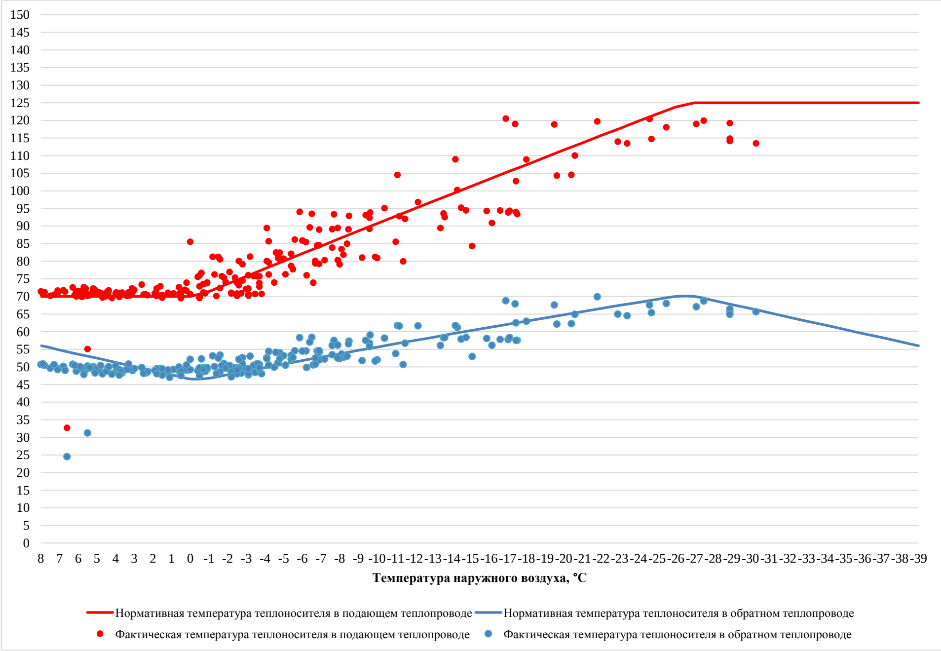
Рисунок 3.12 – Сравнение утвержденного и фактического температурных графиков за 2024 г. – Ильинский тепловывод ЗСТЭЦ
