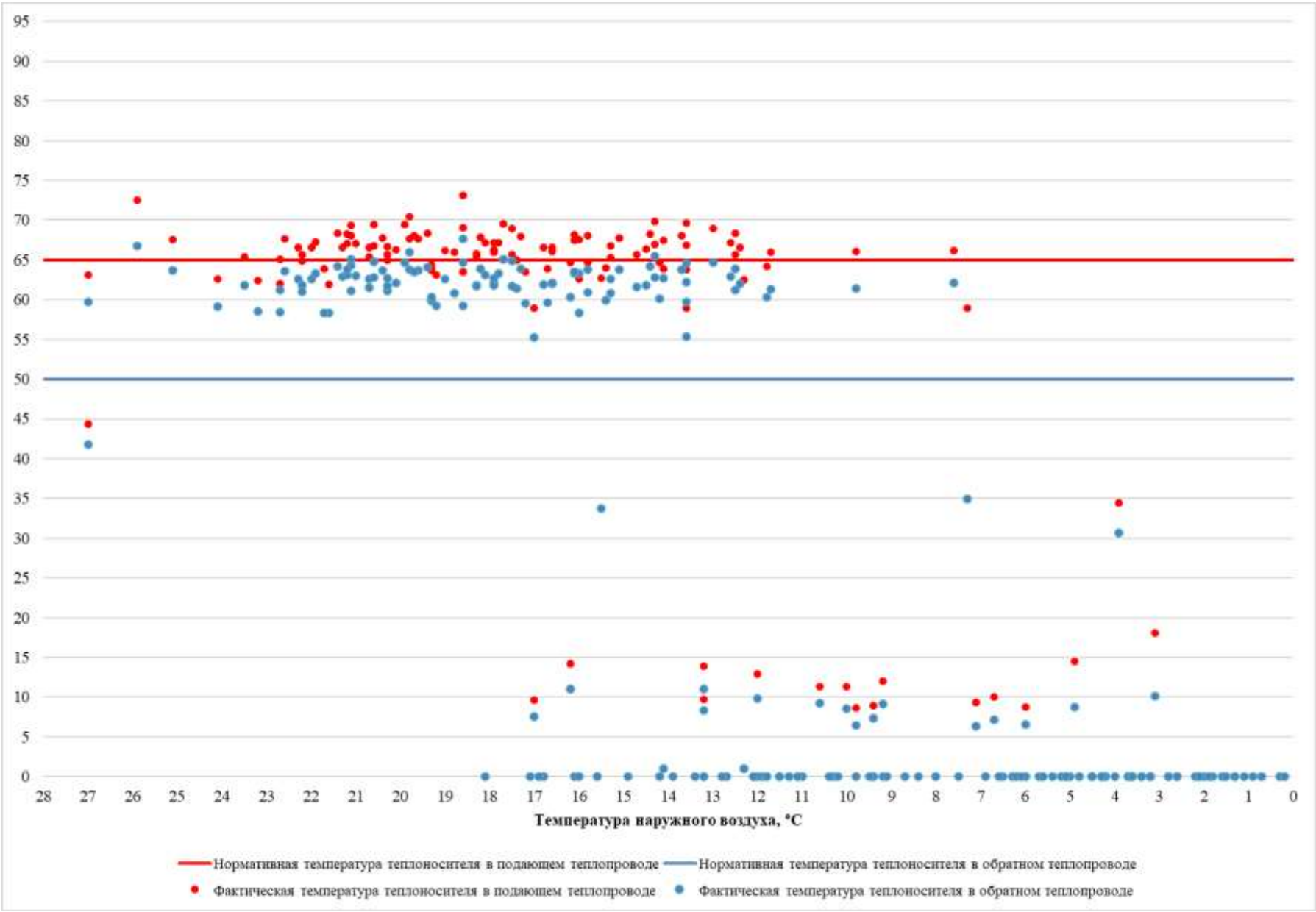
Рисунок 3.41 – Сравнение утвержденного и фактического температурных графиков за 2024 г. – Котельная интерната №66 (Монтажник)
