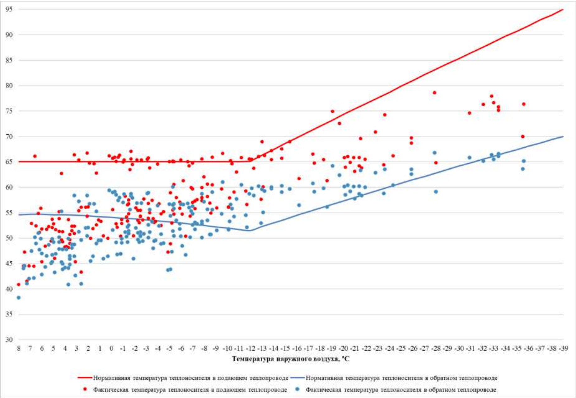
Рисунок 3.37 – Сравнение утвержденного и фактического температурных графиков за 2024 г. – Котельная школы №1
