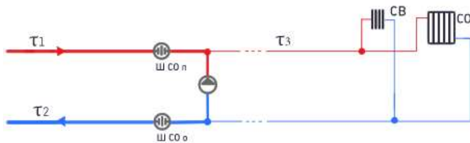
Рисунок 3.8 – ЦТП с насосным присоединением СО
