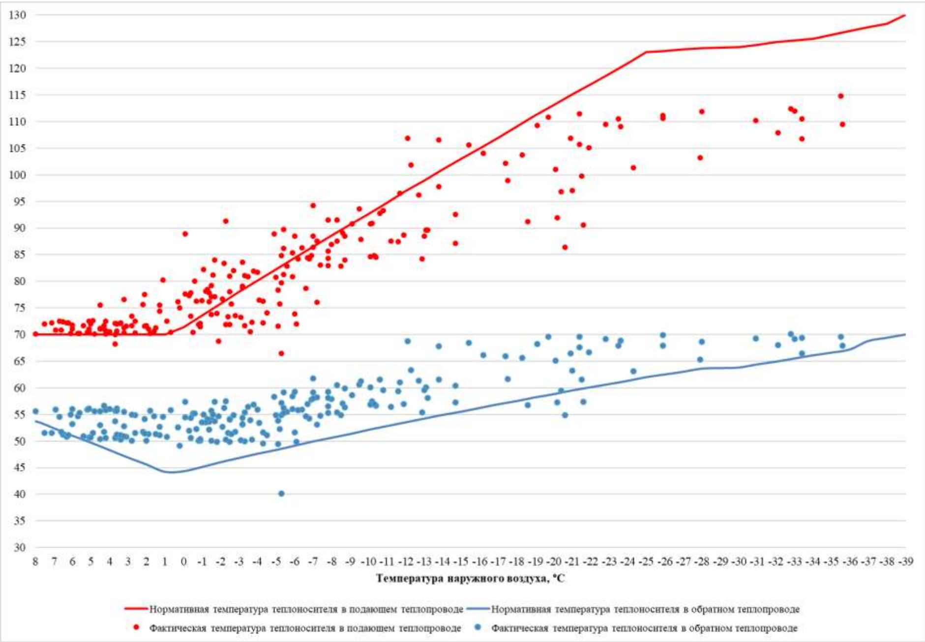
Рисунок 3.17 – Сравнение утвержденного и фактического температурных графиков за 2024 г. – Абашевская районная котельная
