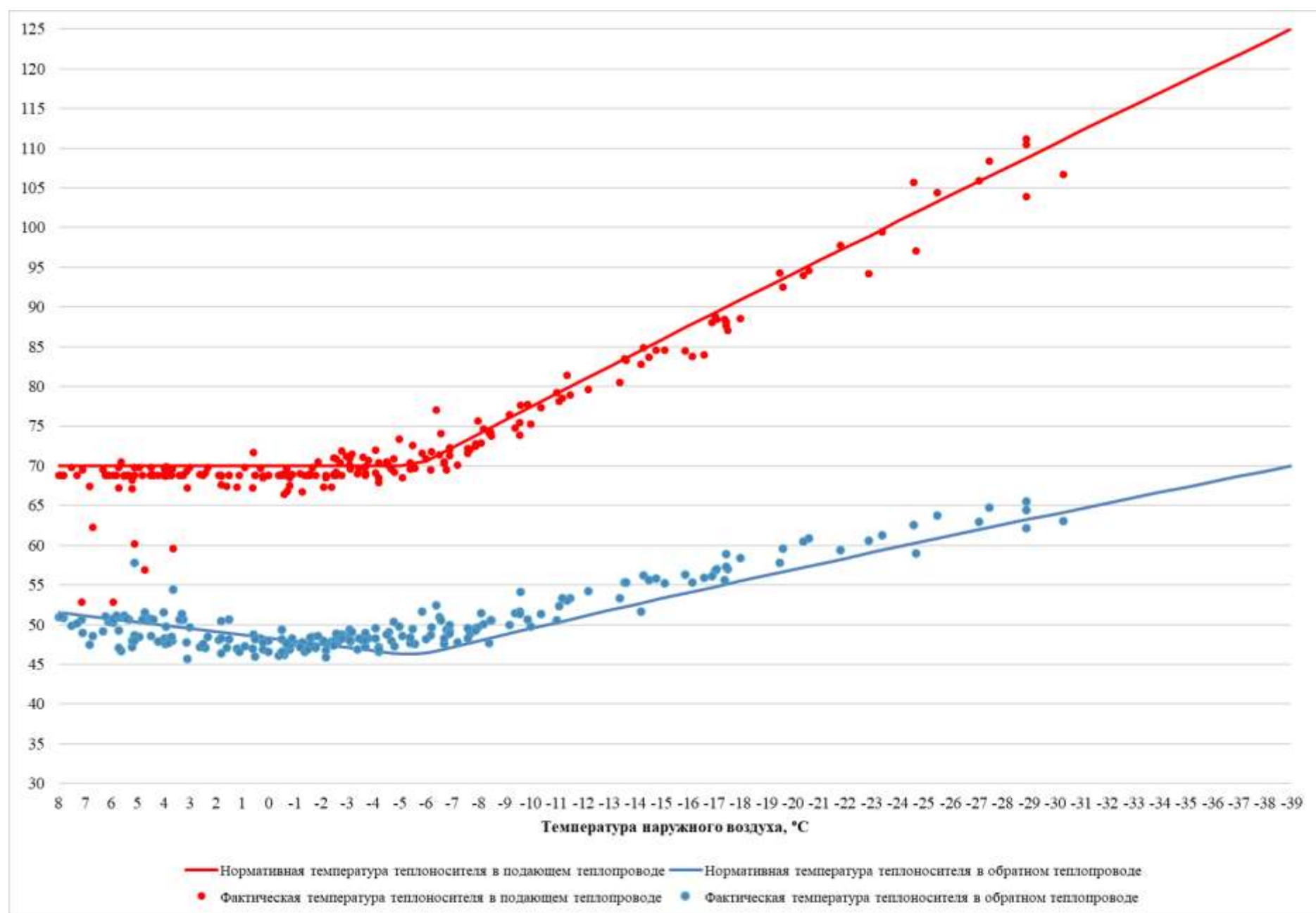
Рисунок 3.16 – Сравнение утвержденного и фактического температурных графиков за 2024 г. – Котельная кв. 24
