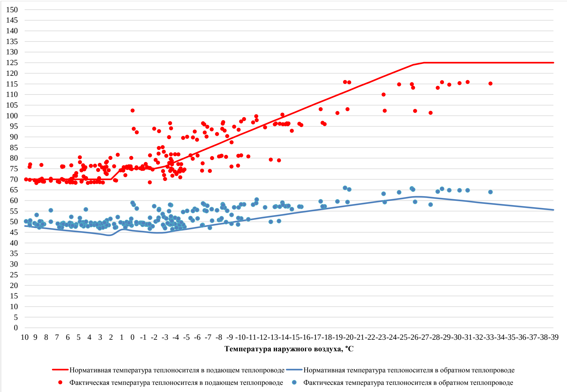
Рисунок 3.13 – Сравнение утвержденного и фактического температурных графиков за 2024 г. – КТЭЦ
