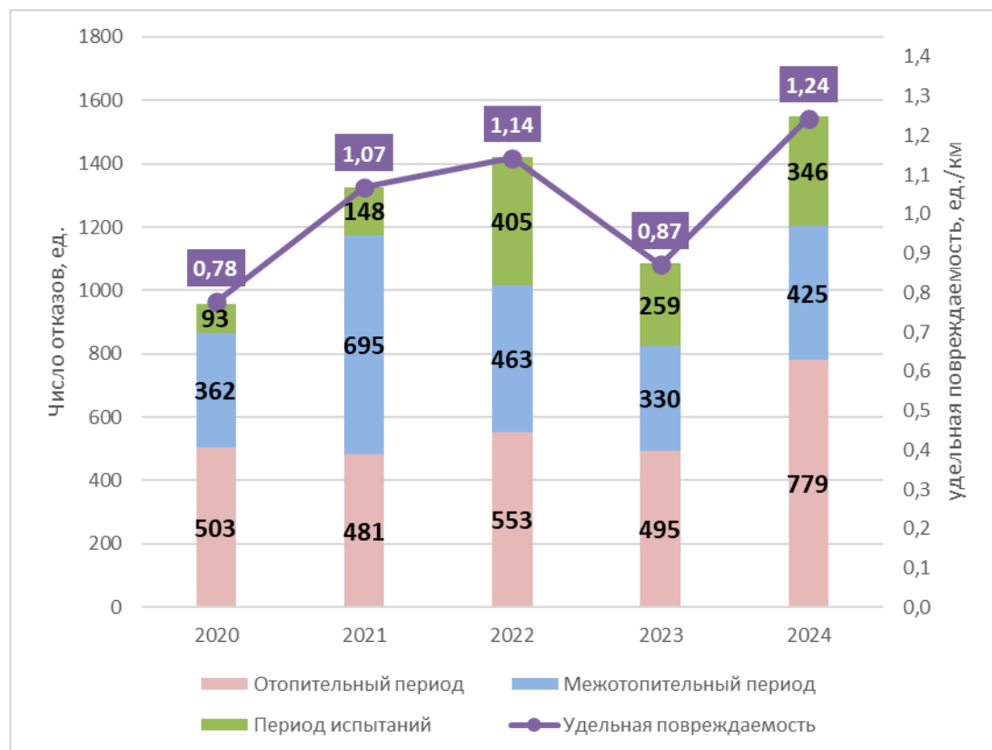
Рисунок 3.48 – Повреждаемость распределительных тепловых сетей и сетей ГВС
