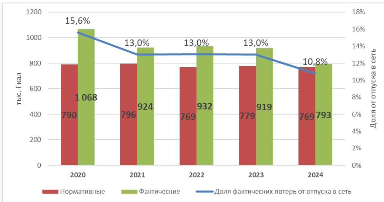
Рисунок 3.51 – Сравнение нормативных и фактических потерь тепловой энергии в тепловых сетях
