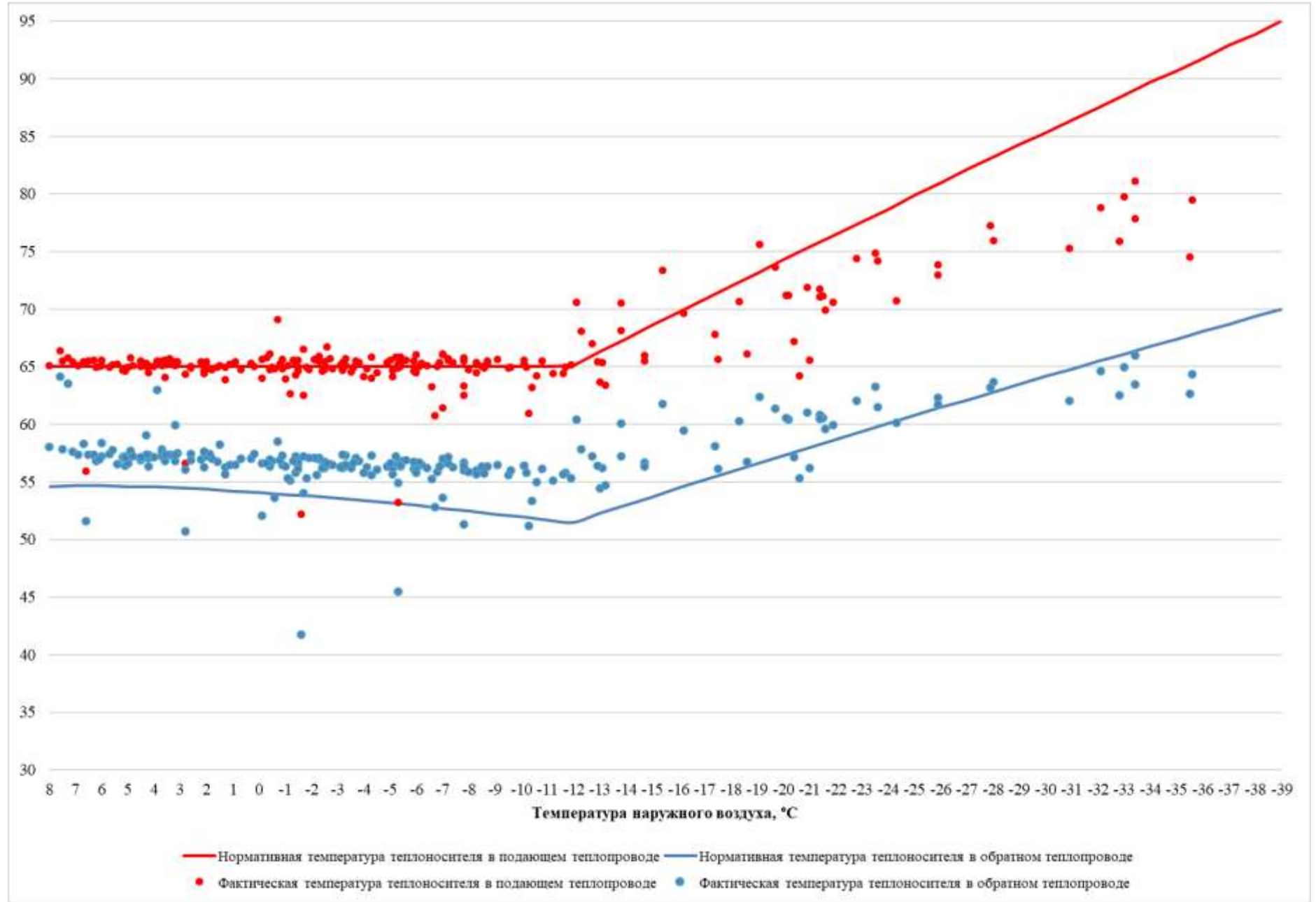
Рисунок 3.18 – Сравнение утвержденного и фактического температурных графиков за 2024 г. – Байдаевская центральная котельная №2
