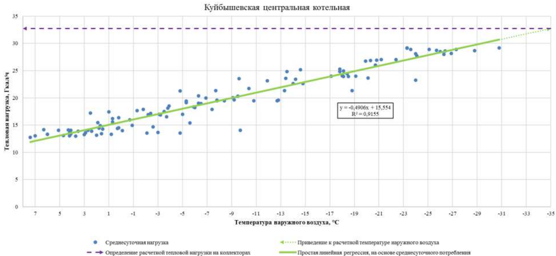
Рисунок 5.12 – Определение расчетной тепловой нагрузки на коллекторах, в зоне действия Куйбышевской центральной котельной
