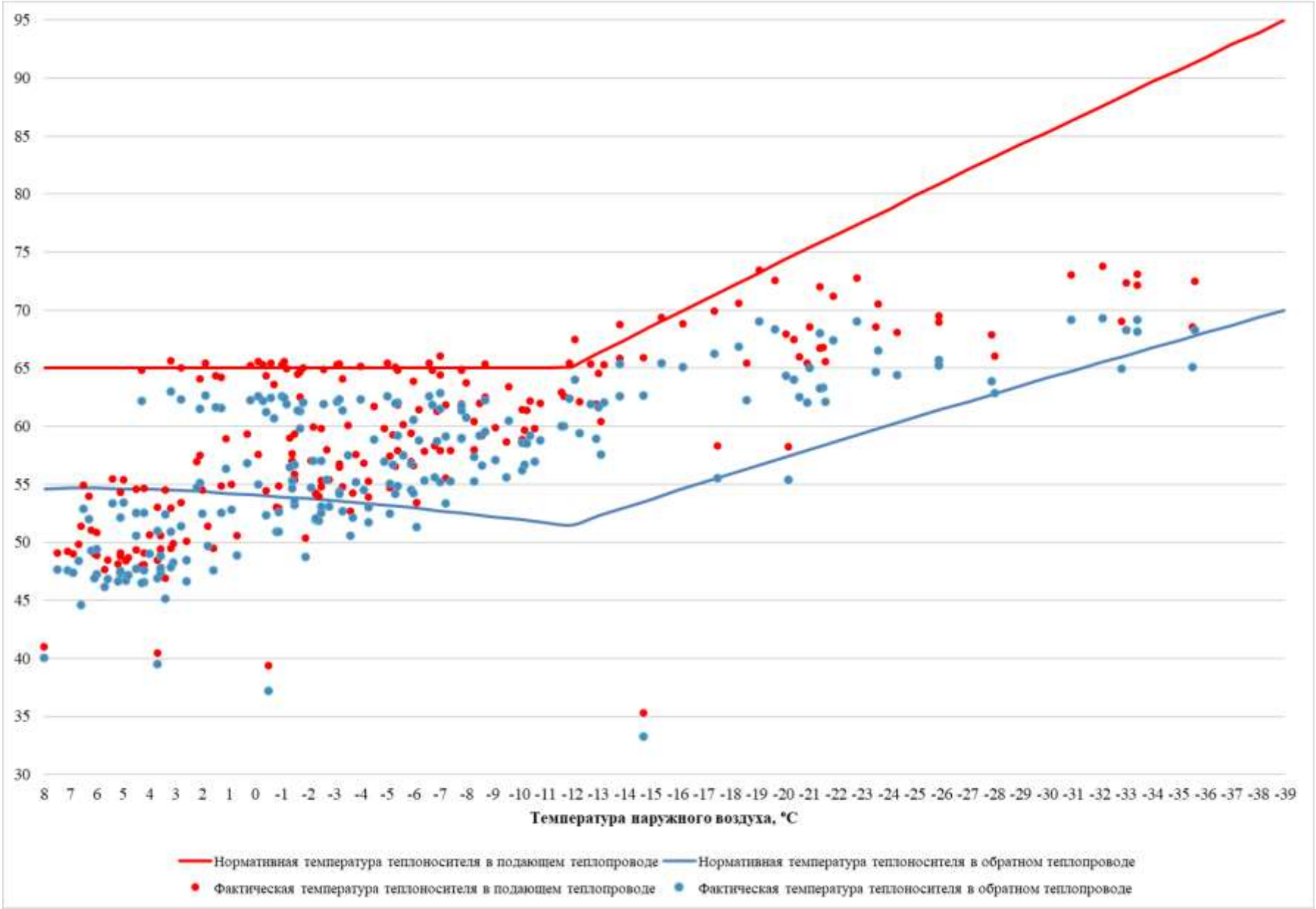
Рисунок 3.42 – Сравнение утвержденного и фактического температурных графиков за 2024 г. – Котельная школы №16
