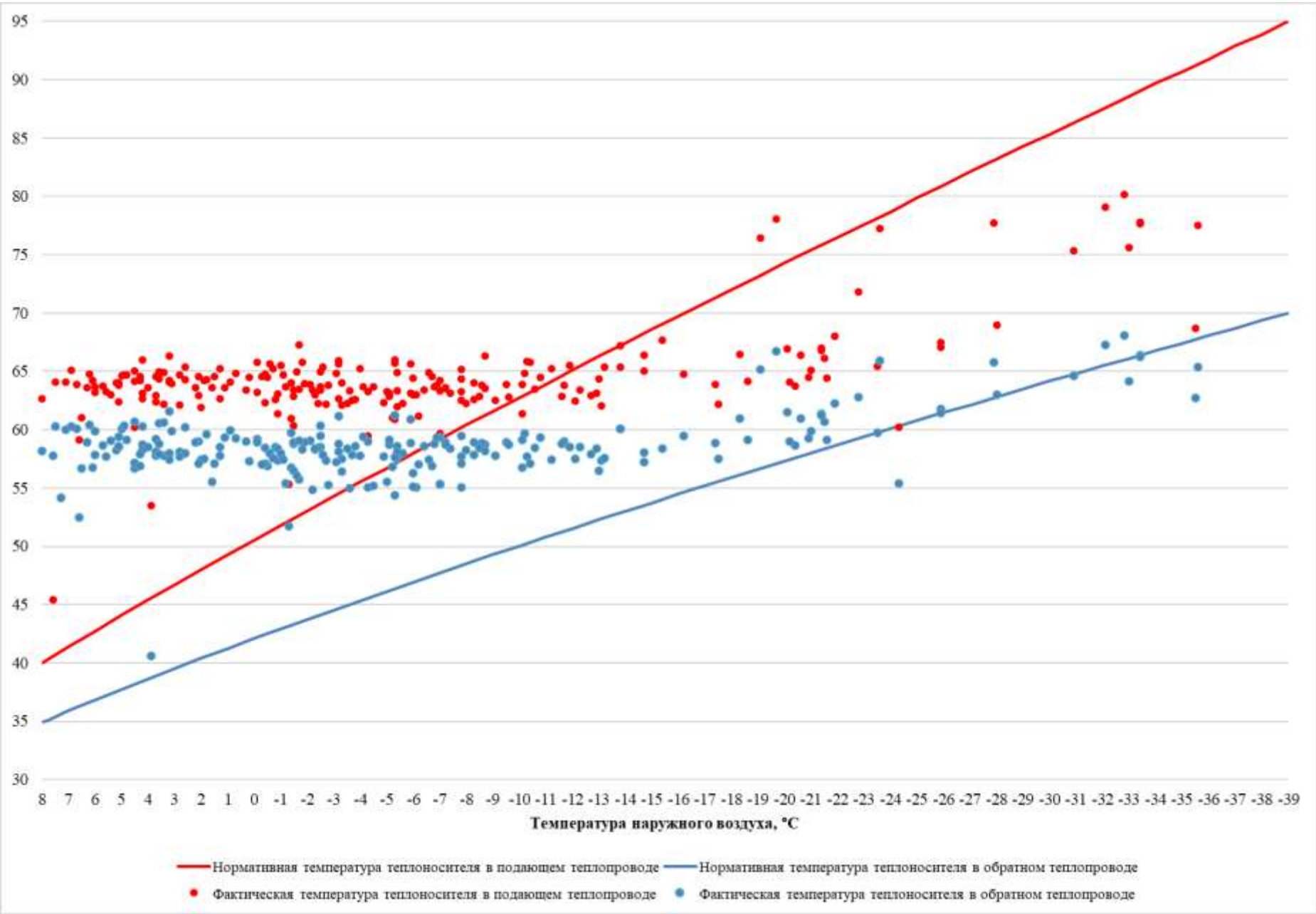
Рисунок 3.44 – Сравнение утвержденного и фактического температурных графиков за 2024 г. – Котельная ст. Полосухино
