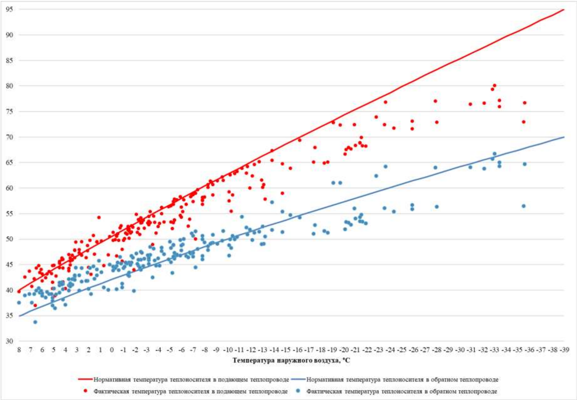
Рисунок 3.43 – Сравнение утвержденного и фактического температурных графиков за 2024 г. – Котельная детского сада №123
