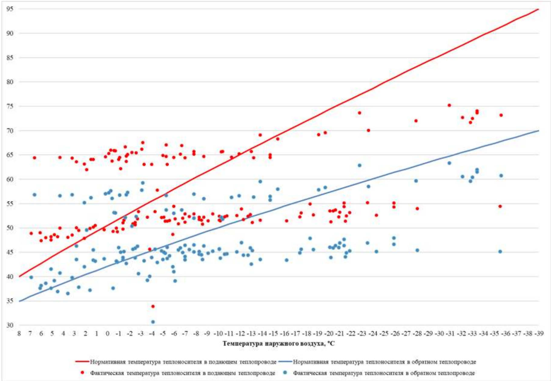
Рисунок 3.39 – Сравнение утвержденного и фактического температурных графиков за 2024 г. – Котельная школы №37
