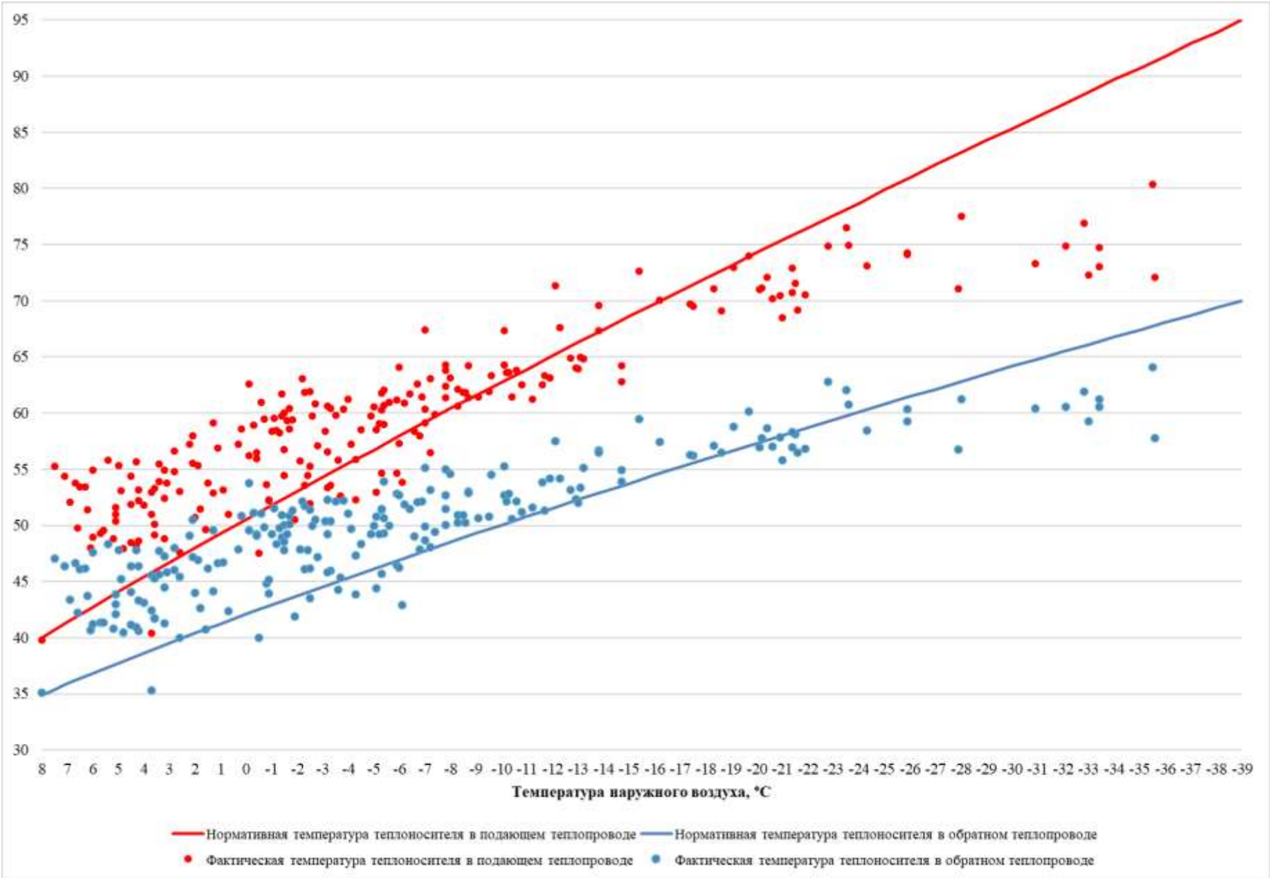
Рисунок 3.32 – Сравнение утвержденного и фактического температурных графиков за 2024 г. – Котельная №1 п. Разъезд-Абагуровский
