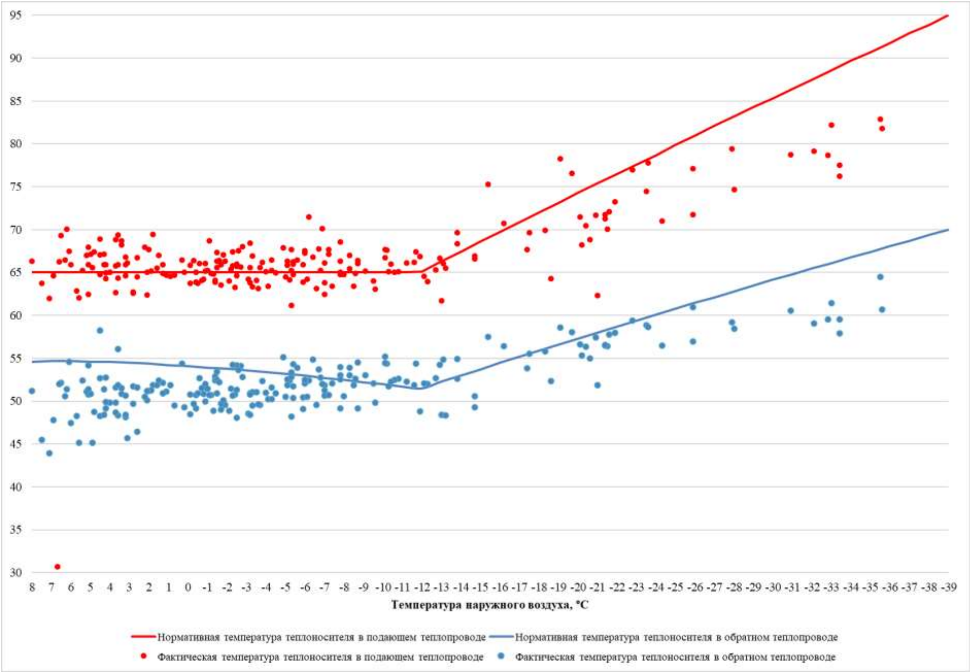
Рисунок 3.24 – Сравнение утвержденного и фактического температурных графиков за 2024 г. – Котельная УПК
