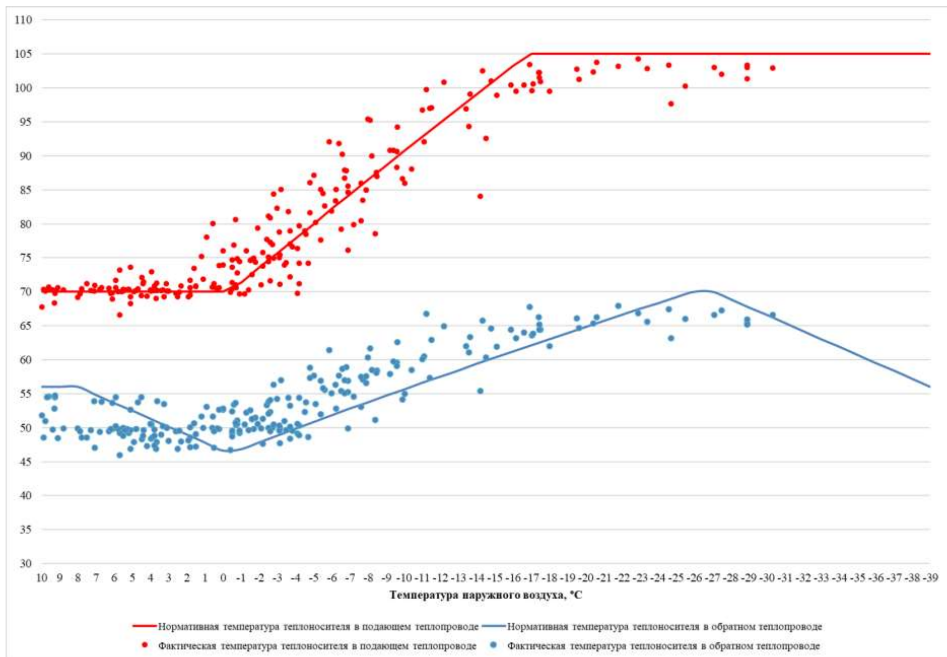
Рисунок 3.15 – Сравнение утвержденного и фактического температурных графиков за 2024 г. – Новоильинская газовая котельная
