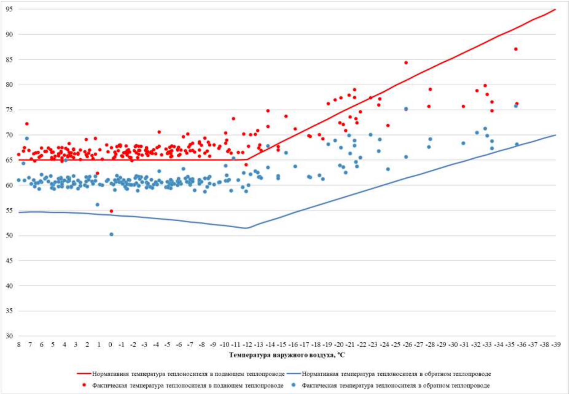
Рисунок 3.35 – Сравнение утвержденного и фактического температурных графиков за 2024 г. – Котельная «РТРС»
