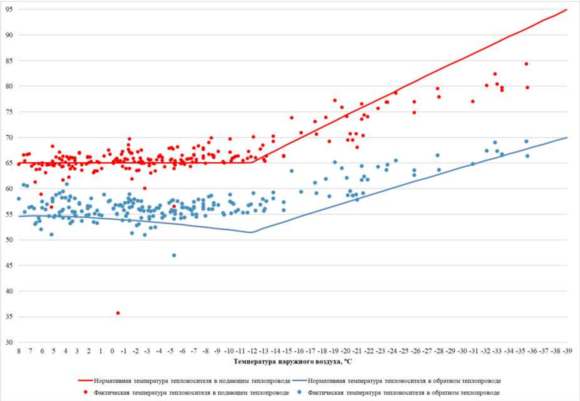
Рисунок 3.25 – Сравнение утвержденного и фактического температурных графиков за 2024 г. – Котельная ОРК «Таргай»
