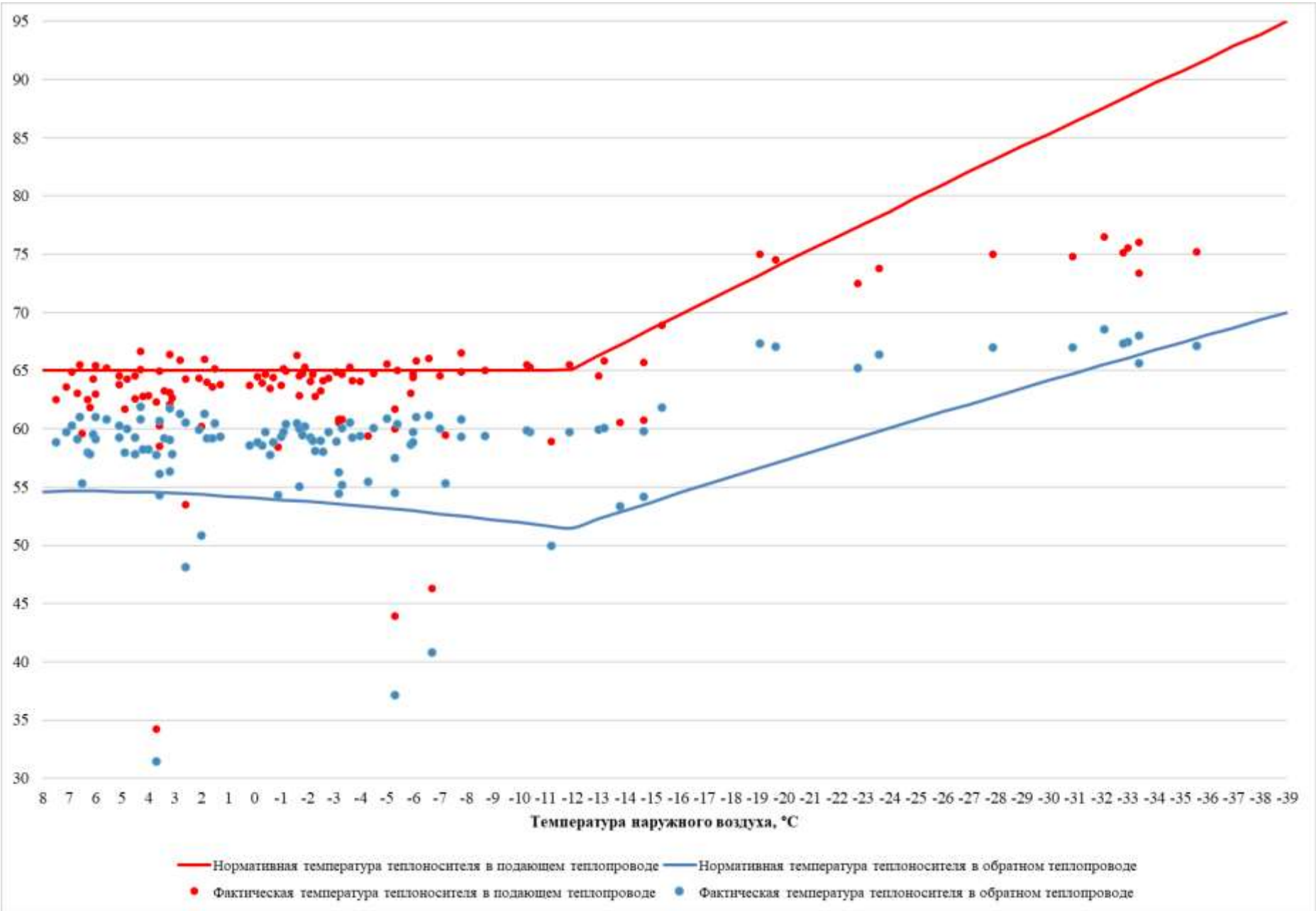
Рисунок 3.36 – Сравнение утвержденного и фактического температурных графиков за 2024 г. – Котельная ОЦ «Голубь»
