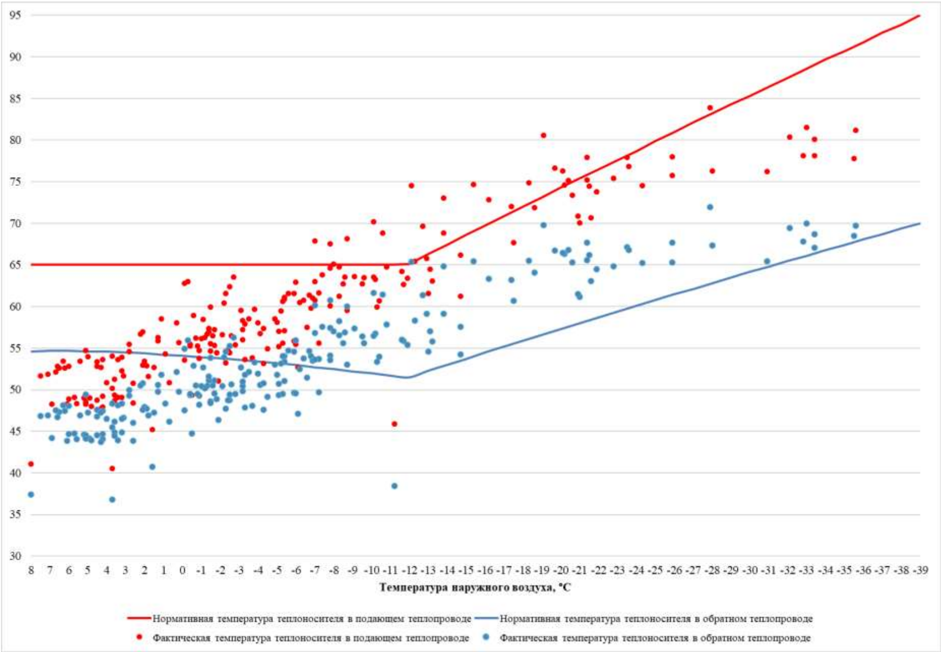
Рисунок 3.27 – Сравнение утвержденного и фактического температурных графиков за 2024 г. – Котельная №2 п. Абагур-Лесной
