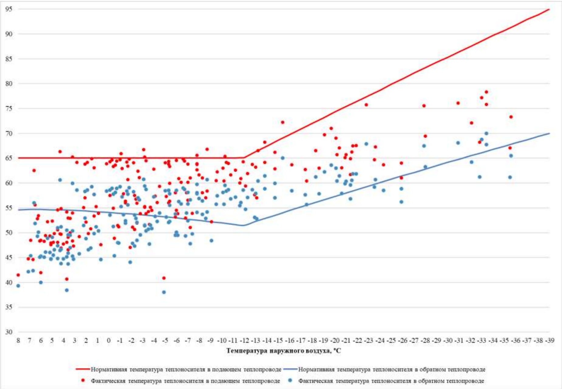
Рисунок 3.38 – Сравнение утвержденного и фактического температурных графиков за 2024 г. – Котельная школы №23
